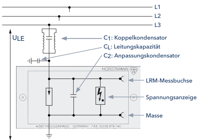
Prinzip des integrierten kapazitiven Spannungsprüfers
